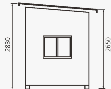
8台尺型立面圖
